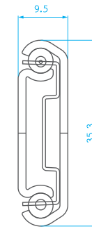
NJ-2000 ( 50lb / 22Kgs )
