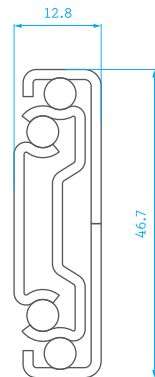
NJ-8000 ( 130lb / 60Kgs )
