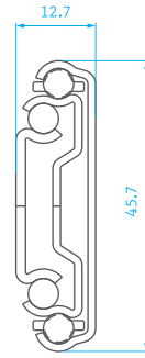
NJ-3J ( 100lb / 45Kgs )
