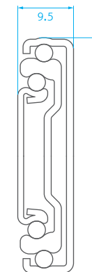
NJ-21A ( 100lb / 45Kgs )
